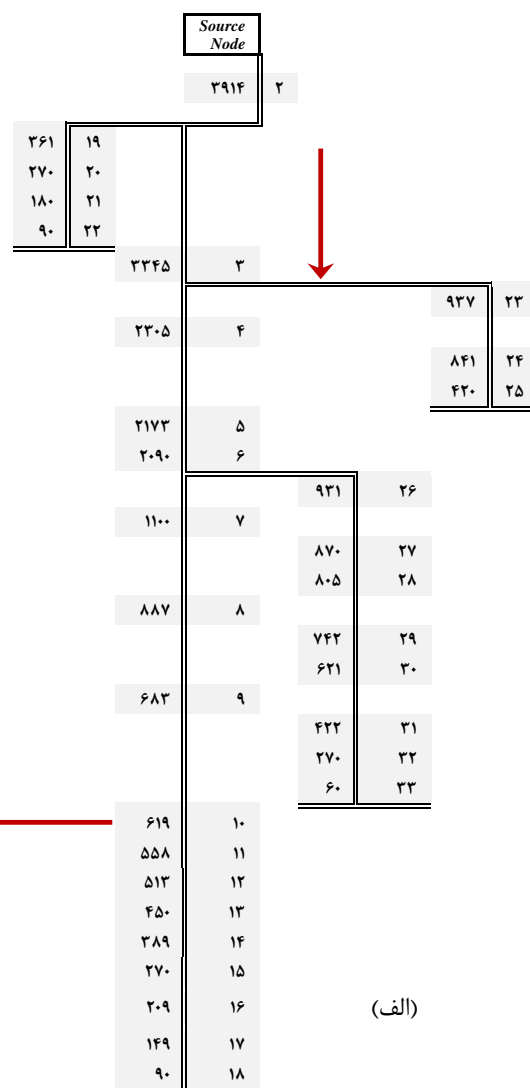
شکل (۲): (الف) نتایج پخش بار برای شبکه ۳۳ با سه وقتی بخش راکتیو بارها حذف شده و بخش اکتیو آن‌ها دو برابر ( 2P_i ) شده است، (ب) مکان بهینه برای تزریق توان اکتیو در بازه‌ی داده شده (از صفر تا ۷۸۲۸/۷ کیلووات)
