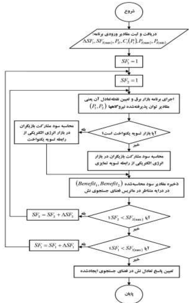
شکل (۵): فلوجارت برنامه تعیین نقطه تعادل نش بازار برق
