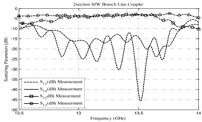
شکل (۱۱): نتایج اندازه‌گیری پیوننده دوبخشی نامتقارن ۳dB ساخته شده
