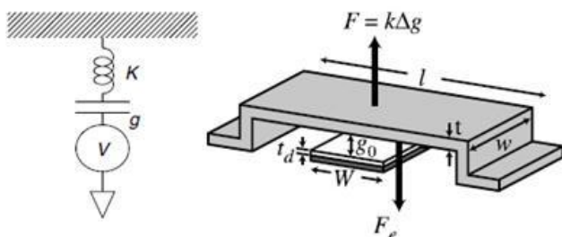
شکل (۳): شماتیک سوئیچ و مدل مکانیکی آن
