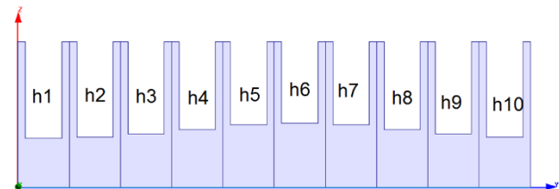
شکل (۴): یک دوره تناوب ساختار دندانه‌ای عمق متغیر و ۱۰ سلول واحد
