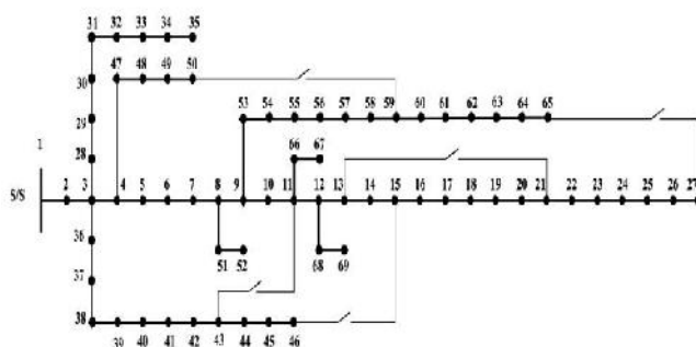
شکل (۶): دیگرام تک خطی شبکه‌ی تست [۳۸].
