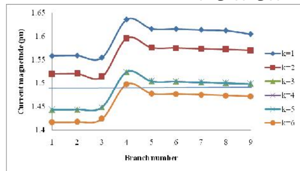
شکل (۷) : روند بهبود منحنی جریان شاخه‌های ۹-۱ در ساعت ۱۷
