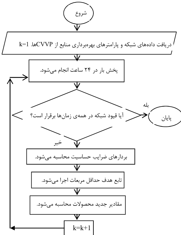
شکل (۴): الگوریتم پیشنهادی برای نیروگاه مجازی فنی.
