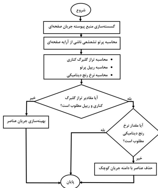
شکل (۳): فلوچارت کلی برای گسسته‌سازی PCCS ها
