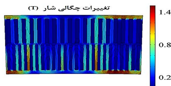
شکل (۱۶): تغییرات چگالی شار بی باری با q=1.5
