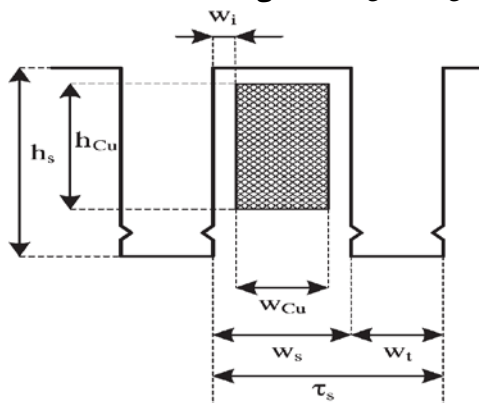
شکل (۱): ابعاد شیار و دندانه
