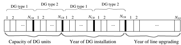
شکل (۱): کدگذاری متغیرهای تصمیم‌گیری مسئله
