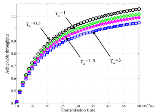
شکل (۹): برون‌دهی برای شبکه کاربران ثانویه برحسب مدت‌زمان
