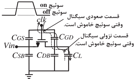
شکل (۵): اثر نفوذ کلاک بر ترانزیستور در حضور خازن پارازیتیک [26] C_{GD}
