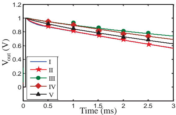
شکل (۱۶): تحلیل گوشه های ولتاژ حالت خاموش کلید پیشنهادی، گوشه (I)، گوشه (II)، گوشه (III)، گوشه (IV)، گوشه (SS)، گوشه (TT)، گوشه (V)
