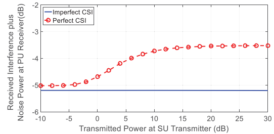
شکل (۷): مقایسه توان سیگنال تداخل بعلاوه نویز دریافتی در مقصد ثانویه با استفاده از روش BF پیشنهادی در حالت ناقص CSI و کامل CSI به ازای R = 8 و L = 2
