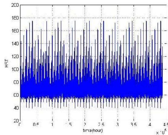
شکل (۸): نمودار دمای نقطه داغ ترانسفورمر برای بارگذاری سبک
