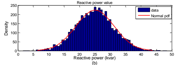
شکل (۳): تابع توزیع احتمالی توان‌های مصرفی در باس ۲۷
