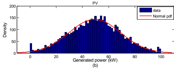
شکل (۴): تابع توزیع احتمالی توان‌های تولیدی
