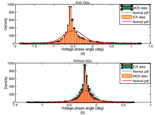
شکل (۷): تابع توزیع احتمالی زاویه فاز ولتاژ باس ۲۷ در دو سناریو (a): زاویه فاز ولتاژ باس ۲۷ در حضور تولیدات پراکنده. (b): زاویه فاز ولتاژ باس ۲۷ بدون تولیدات پراکنده
