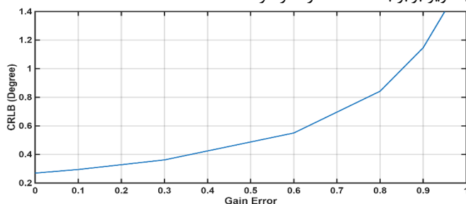
شکل (۹): مقدار CRLB(\theta) بر حسب مقادیر مختلف خطای بهره
