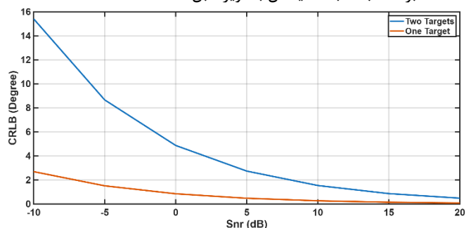
شکل (۶): مقدار CRLB(\theta) برای حالت بهینه با تعداد اهداف مختلف بر حسب نسبت سیگنال به نویز
