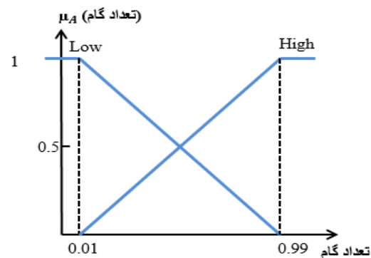
شکل (۵): توابع عضویت برای متغیرهای ورودی تعداد گام
