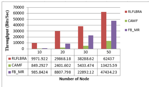
شکل (۱۰): نرخ گذردهی
