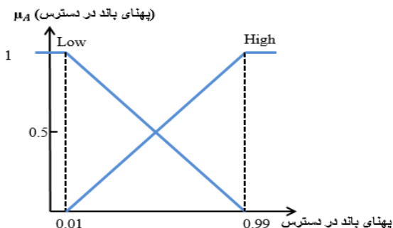
شکل (۴): توابع عضویت برای متغیرهای ورودی پهنای باند
