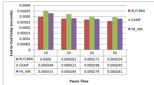
شکل (۹): تأخیر انتها به انتها
