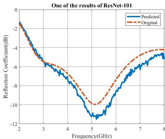
شکل (۲-۸): نتیجه مقایسه داده اصلی (اولین داده اعتبارسنجی) با تخمین شبکه رزنت-۱۰۱ (گام دوم)
