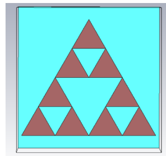
شکل (۲-۳): نمای جلویی جاذب طراحی شده
