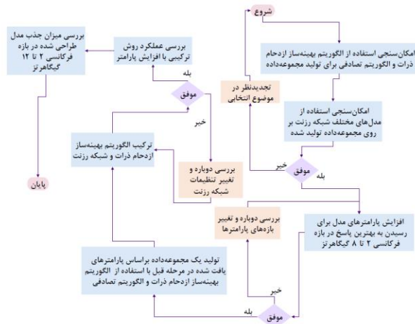
شکل (۱-۱): روندنمای کلی مسیر مقاله
