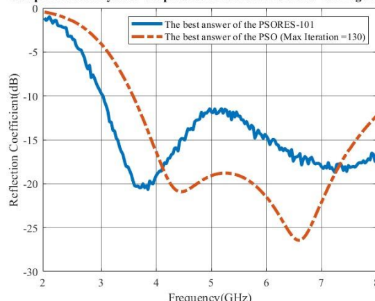
شکل (۲-۱۰): مقایسه خروجی بهینه یافت شده توسط الگوریتم PSO و روش ترکیبی
