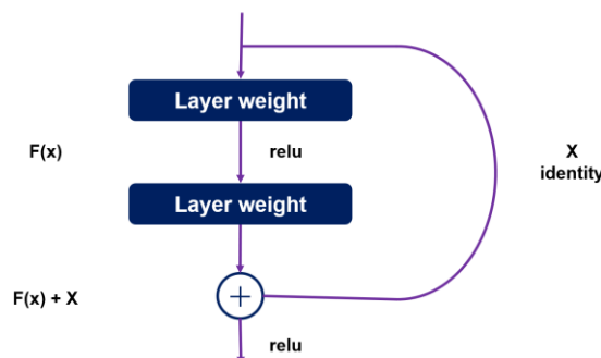
شکل (۲-۴): نمونه یک بلوک Residual
