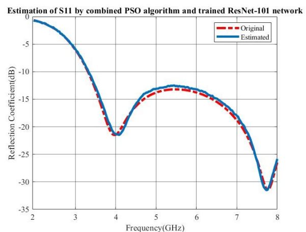
شکل (۲-۷): نتیجه تخمین و یافتن پاسخ بهینه توسط روش ترکیبی
