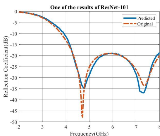
شکل (۲-۶): نتیجه مقایسه داده اصلی (اولین داده اعتبارسنجی) با تخمین شبکه رزنت-۱۰۱ (گام اول)
