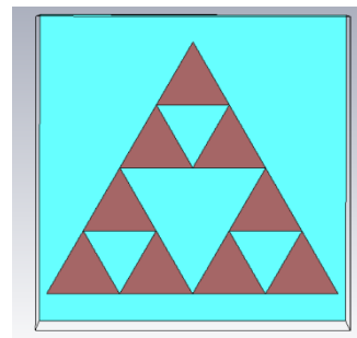
شکل (۲-۳): نمای جلویی جاذب طراحی شده
