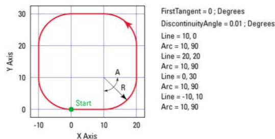
شکل (پ-۱): نمونه‌ای از کد مورد نیاز برای توضیح یک مسیر ساده به روش خط و قوس
