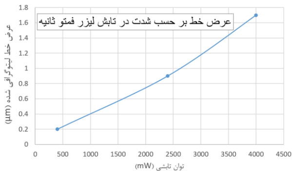
شکل (۴): عرض خط لیتوگرافی شده در اثر تابش لیزر پالس کوتاه فمتوثانیه در توان‌های تابشی متفاوت
