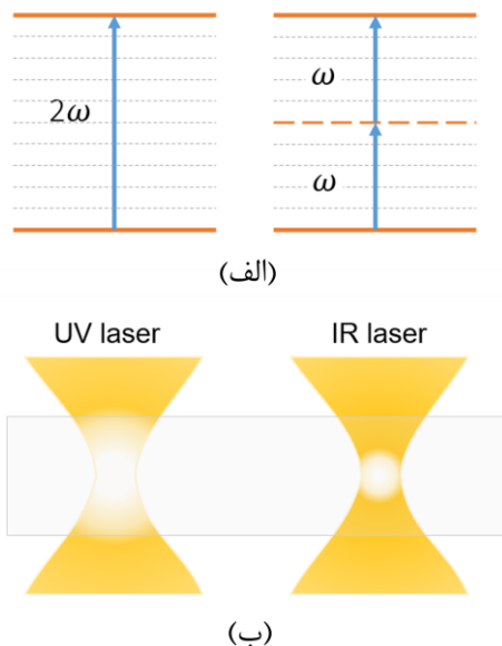
شکل (۲): (الف) نمودار تراز های انرژی در فرآیند جذب معمولی و جذب دوفوتونی، (ب) باریکهی فوکوس شدهی لیزر برای دو حالت لیزر UV معمولی و لیزر فمتو ثانیه IR
