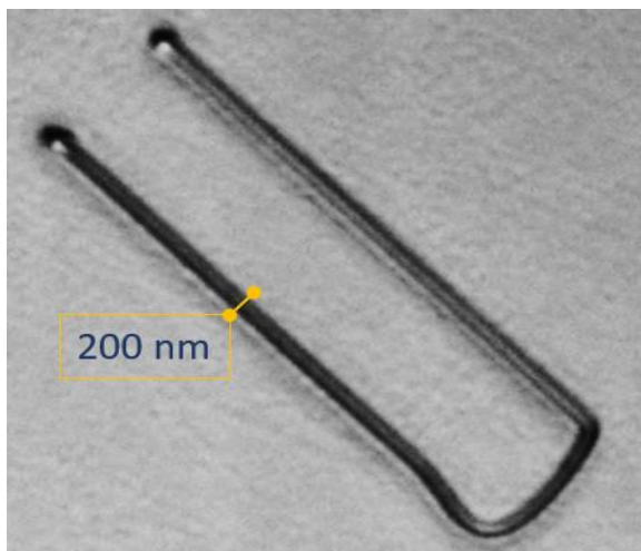
شکل (۶): نانوساختار تولیدشده با استفاده از لیتوگرافی جذب دوفوتونی توسط لیزر فمتوثانیه
