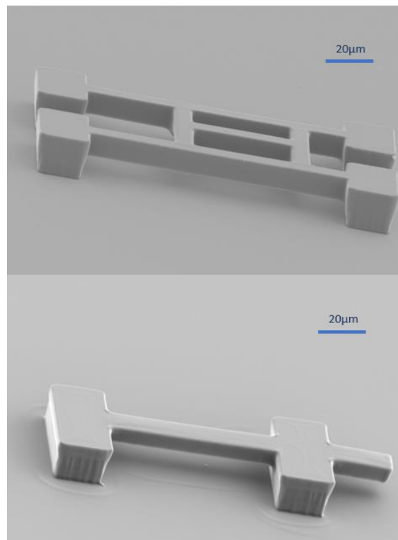
شکل (۹): نمونه‌ای از ریزساختار سه‌بعدی تهیه‌شده به روش لیتوگرافی جذب دوفوتونی
