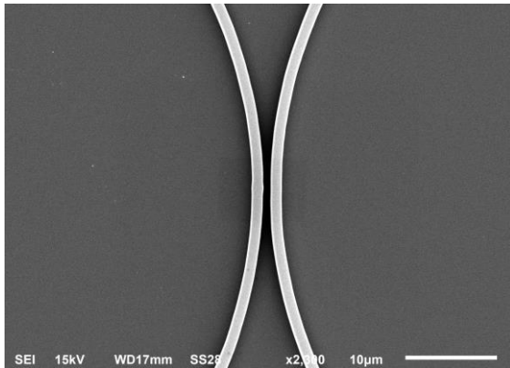
شکل (۸): نمای بزرگ نمایی شده حفره میان ریز حلقه ها که دقت، ظرفیت ساخت و صافی سطح دیواره ها را نشان می دهد
