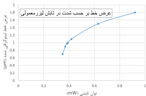
شکل (۳): عرض خط لیتوگرافی شده در اثر تابش لیزر پیوسته معمولی در توان‌های تابشی متفاوت
