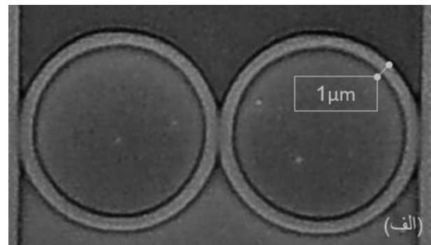
شکل (۸): نمای بزرگ نمایی شده حفره میان ریز حلقه ها که دقت، ظرفیت ساخت و صافی سطح دیواره ها را نشان می دهد
