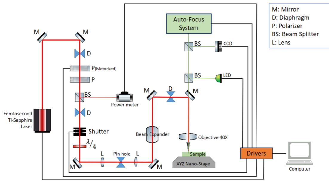
شکل (۵): چیدمان آزمایشگاهی لیتوگرافی جذب دو فوتونی با لیزر فمتوثانیه در آزمایشگاه مدارهای مجتمع نوری
