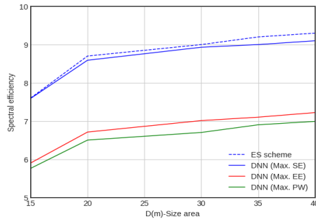
شکل (۶-ا): راندمان طیفی نسبت به مساحت (D)
