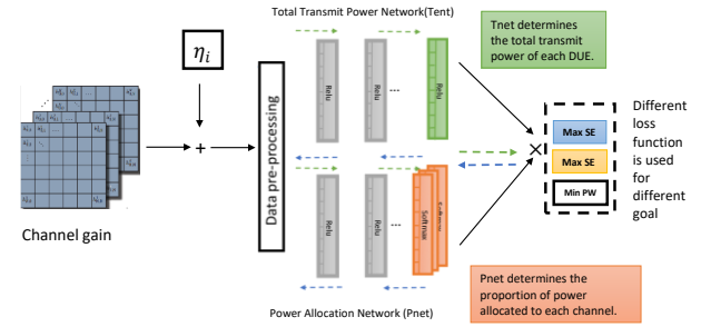
شکل (۳): تخصیص منبع مبتنی DNN تحت قید نقیصه‌های سخت‌افزاری
