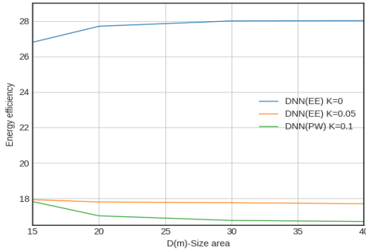
شکل ۸(b): بهره‌وری انرژی نسبت به مساحت (D)
