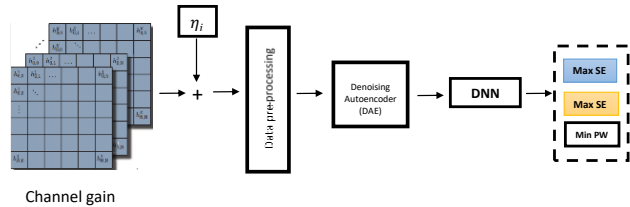
شکل (۵): مدل سیستم با DAE
