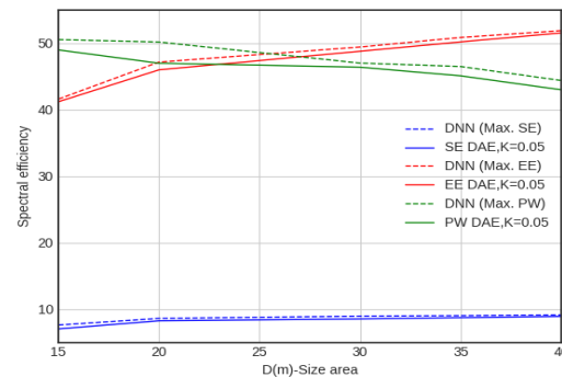
شکل (۹): نتایج RA هنگام استفاده از DAE
