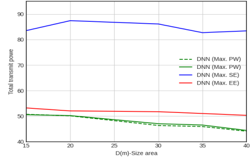
شکل ۸(d): کل توان انتقالی نسبت به مساحت (D)
