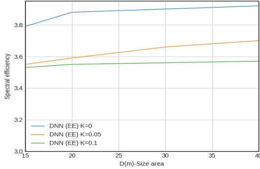
شکل ۸(a): کارایی طیفی نسبت به مساحت (D)
