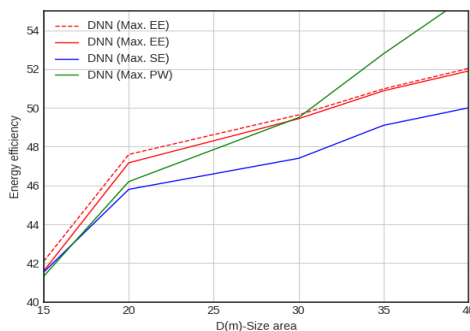
شکل (۶-ب): بهره‌وری انرژی نسبت به مساحت (D)
