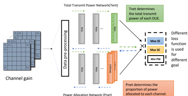
شکل (۲): تخصیص منابع مبتنی DNN در غیاب نقیصه‌های سخت‌افزاری
